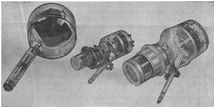
Передающие трубки типа иконоскоп (слева) и су- периконоскоп
