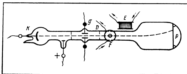
Трубка Рентгена
