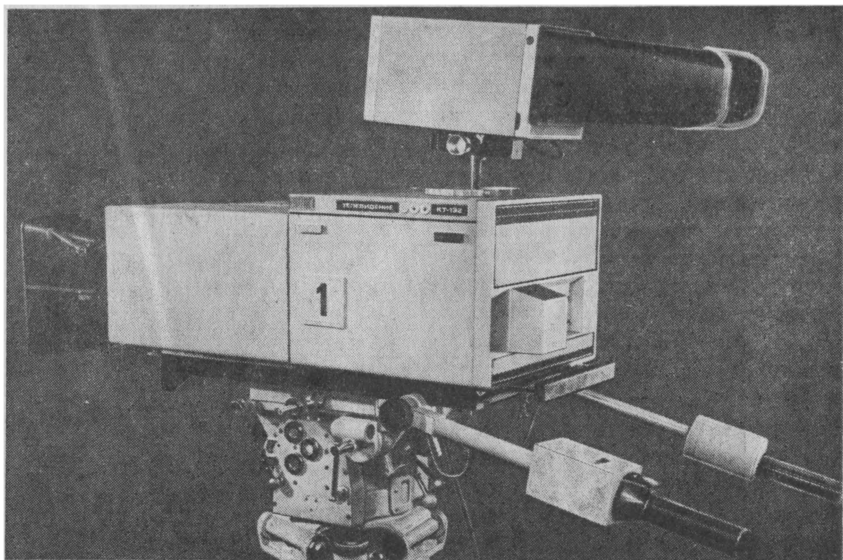
Передающая ТВ камера КТ-132
