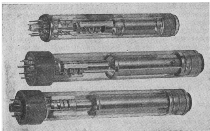
Глетиконы — передающие трубки для цветного телевидения
