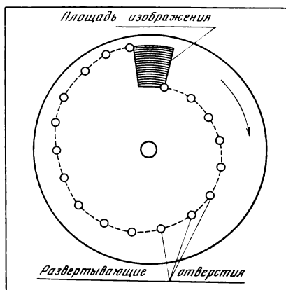
Диск Нипкова
