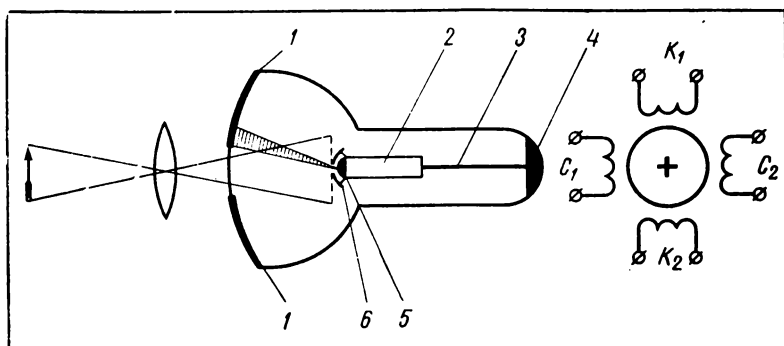
Оптический диссектор Б. А. Рчеулова
