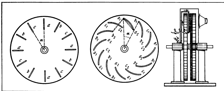
Светораспределитель А. А. Полумордвинова
