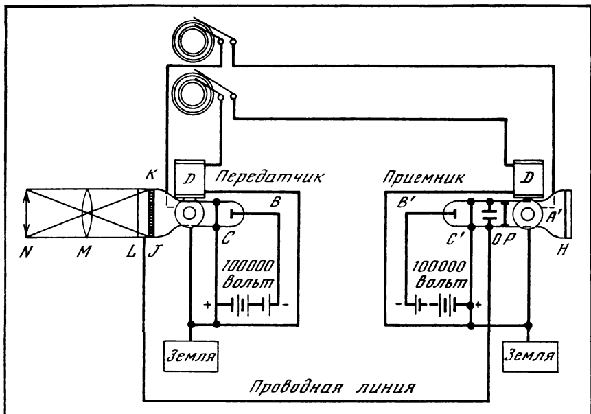
Схема А. К. Суинтона
