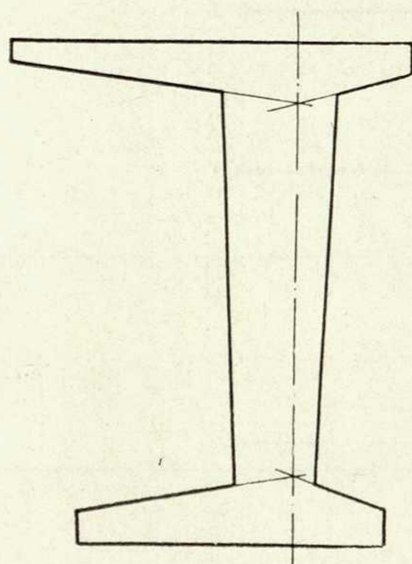
10. Принципиальная схема построения формы стойки.
