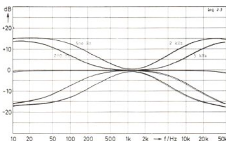
2.3 Frequenzgang Klangsteller (Mittenposition) halb und voll angehoben bzw. abgesenkt
