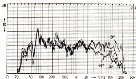
3 Rundstrahlverhalten für die Hörwinkel 0, 20 und 40°, Kurven übereinandergeschrieben
