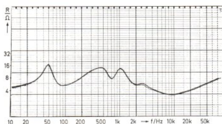
3 Impedanzkurve im Bereich 10 Hz bis 50 kHz
