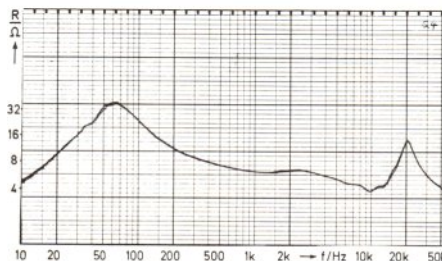
4 Impedanzverlauf im Bereich 10 Hz bis 50 kHz, gemessen an beiden Exemplaren bei einer Leistung von 5,6 mW an 4 \Omega . Die kleinste Impedanz tritt bei 9,5 kHz auf und beträgt dort 3,8 \Omega . Die ESL 63 sind nach DIN als 4- \Omega -Boxen zu betrachten.
