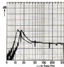
5 Tiefenresonanz des Tonarms mit dem Tonabnehmer Stanton 680 SL: lateral ca. 12 Hz, vertikal 16 Hz
