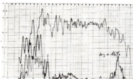
5 Schalldruckkurve, k_2 und k_3 der Quad-Elektrostaten aus dem Jahre 1969 bei 85 DIN-Phon, Mikrofon in 2 m Abstand auf Achse
