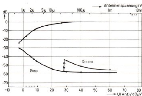
5 Signal-Rauschspannungs-Diagramm des CE 16
