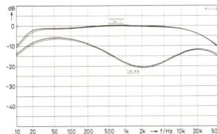
1.2 Frequenzgang Laut-Leise-Schaltung
