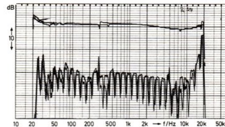
6 Frequenzgang und Übersprechen des eingebauten Tonabnehmers Stanton 680 SL
