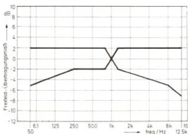
2 Toleranzfeld der Sollkurve des Freifeld-Übertragungsmaßes bei Kopfhörern nach DIN 45 500
