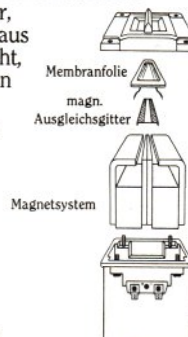
Prinzip des Bändchen Hohtöners
