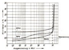
2 Klirrgang im linken Kanal, gemessen bei drei Frequenzen über der Ausgangsleistung; entnommen dem Testbericht in HiFi-Stereophonie 5/63
