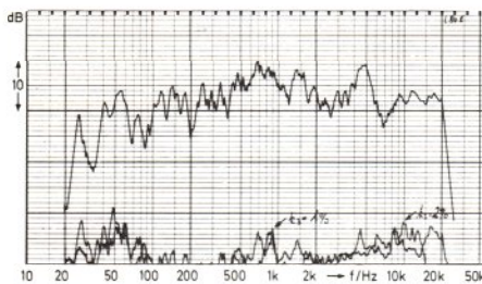
8 Wie Bild 7, gemessen an einem zweiten Exemplar
