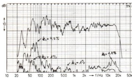
1 Schalldruckkurven und harmonische Verzerrungen k_2 und k_3
