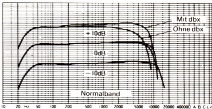
Gesamtfrequenzumfang RS-M 270 X (Klirrfaktor 3%)
