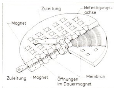
1 Prinzip des orthodynamischen Kopfhörers (nach Yamaha)
