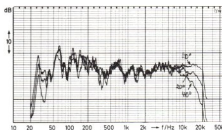
2 Rundstrahlverhalten für die Hörwinkel 0, 20, 40°
