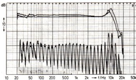
6 Frequenzgang und Übersprechen mit dem eingebauten Shure-Tonabnehmer
