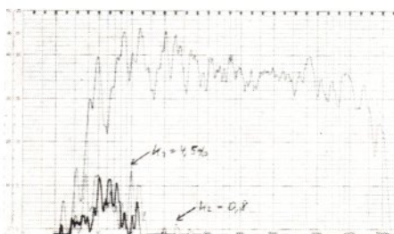
6 Schalldruckkurve, k_2 und k_3 der Quad-Elektrostaten aus dem Jahre 1969 bei 75 DIN-Phon, Mikrofon in 2 m Abstand
