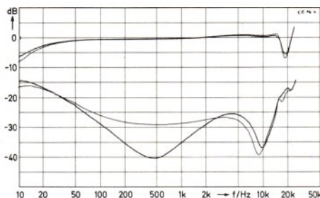
4 Frequenzgang und Übersprechen des Braun CE 16
